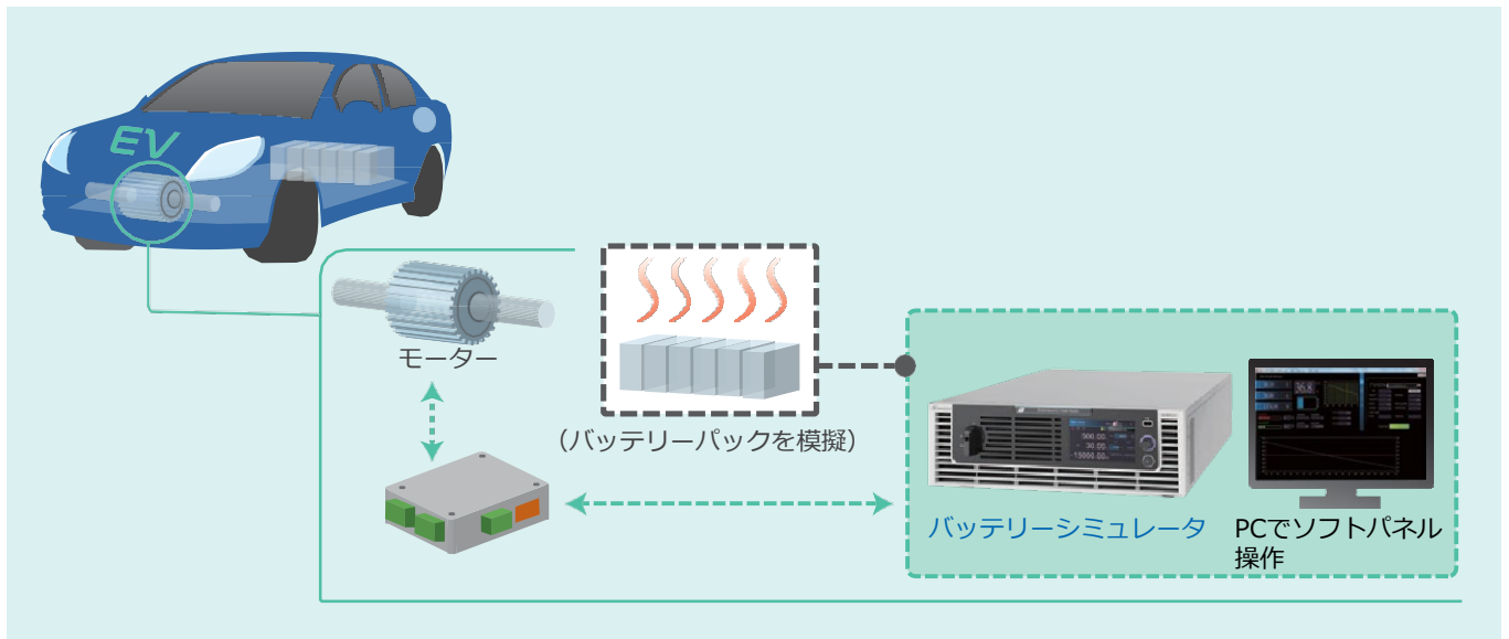
自動車起動システム モータードライバテストアプリケーション
