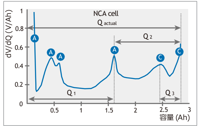
dV/dQ 曲線
