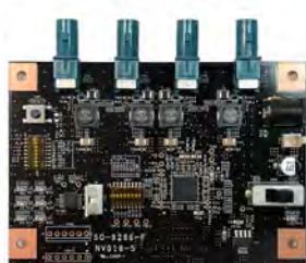
GMI-9286-F (Maxim MAX9286搭載)
