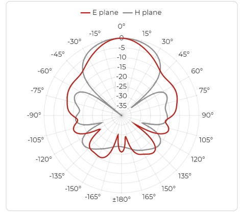
Port B, 6 GHz
