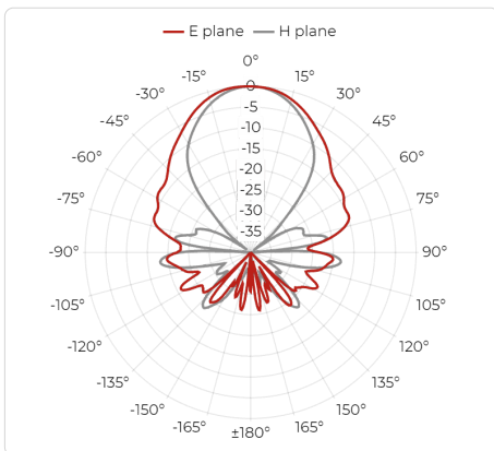
Port B, 14 GHz
