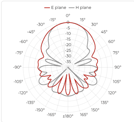
Port B, 8 GHz
