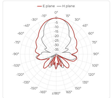
Port B, 12 GHz
