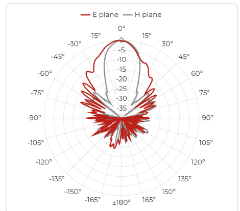
Port B, 18 GHz
