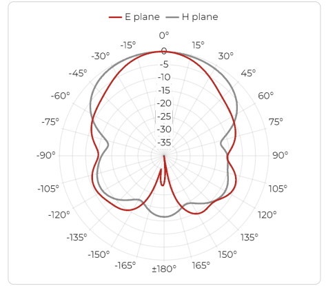
Port B, 2.4 GHz
