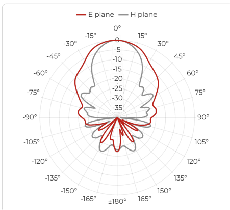
Port B, 4.8 GHz
