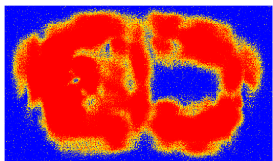
非接触空中超音波検査によるCスコープ画像
