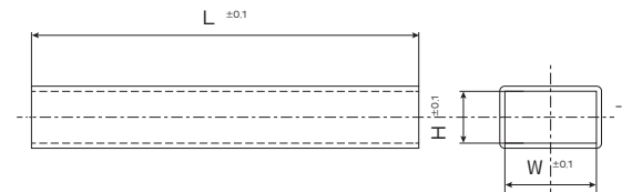
IFM6 貫通管
