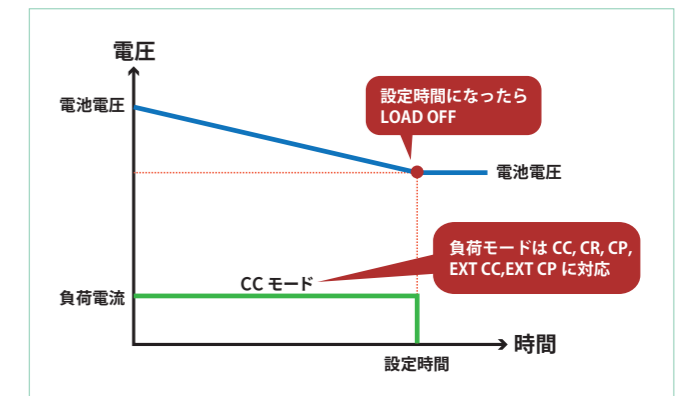
放電時間設定時の動作イメージ(CCモードの場合)
