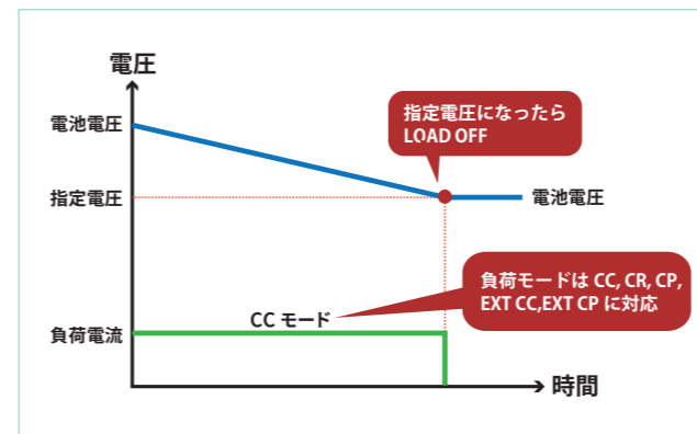
指定電圧設定時の動作イメージ(CCモードの場合)
