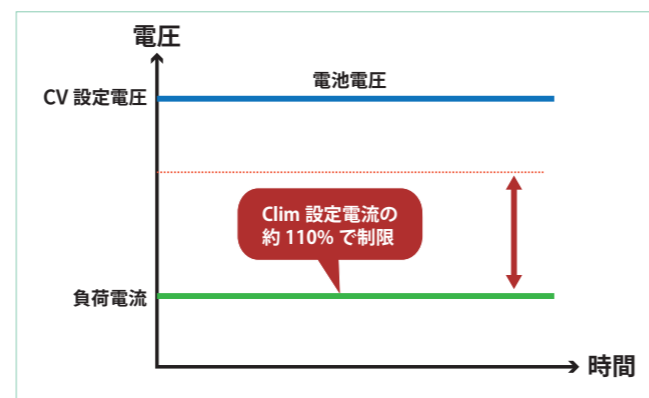
放電時の動作イメージ (CV+Clim 動作)
