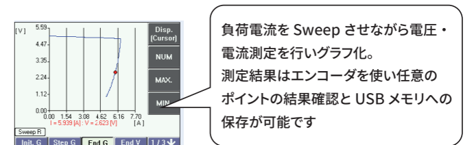
Sweep CRモード実行例(例:過電流特性試験)
