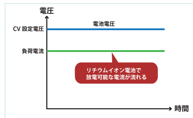
放電時の動作イメージ (従来の CV 動作)
