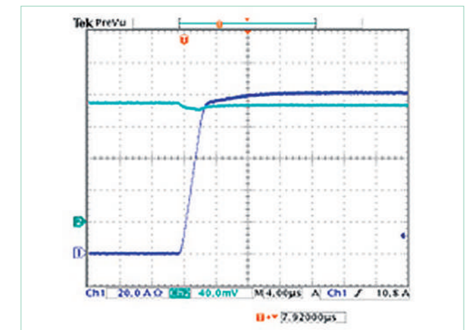
なめらかな電流応答を実現
