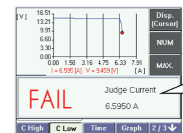
Sweep CRモード判定例(例:過電流特性試験)
