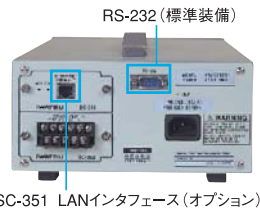
SC-351 LANインターフェース (オプション)
