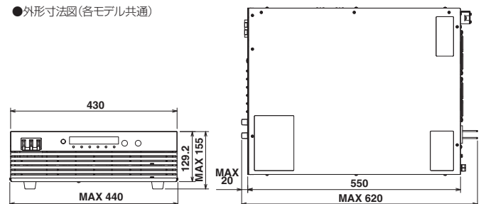
●外形寸法図 (各モデル共通)
