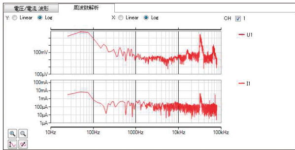
高次高調波周波数解析の画面例
