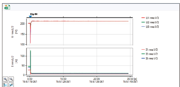
電圧降下の画面例 (30 秒イベント変動データ)
