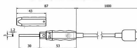
水平型 (Transverse): PA-400T
